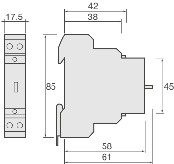
Габаритні розміри Імпульсне реле
