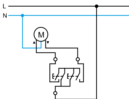
Управління жалюзі за допомогою клапового перемикача без фіксації з ел. блокуванням (схема при використанні клапового перемикача з фіксацією аналогічна)
