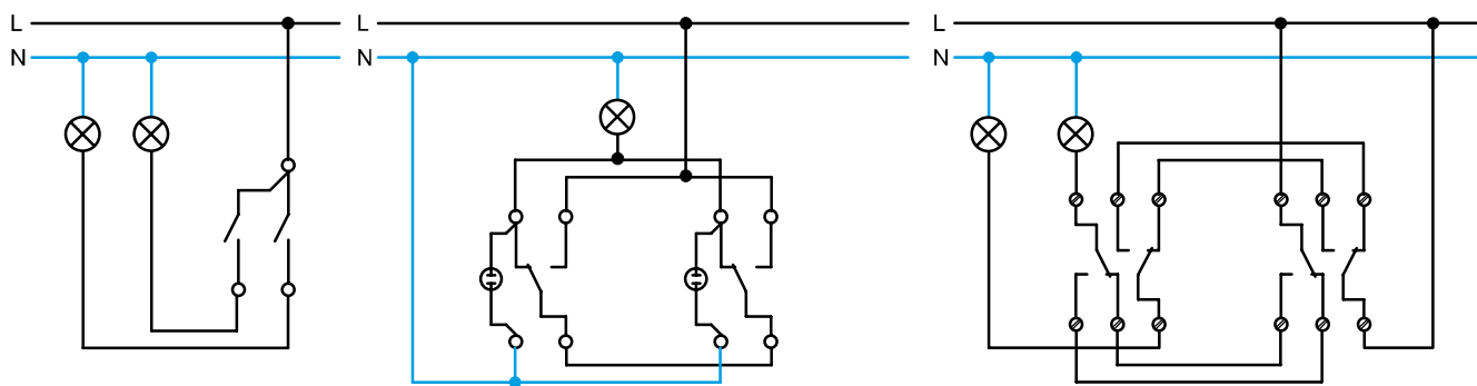
Вимикач двоклавішний
