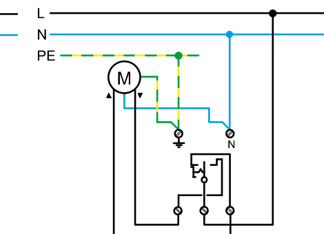
Управління жалюзі за допомогою клапового перемикача (з фіксацією) з мех. блокуванням з використанням затисків N і PE (схема при використанні клапового перемикача без фіксації аналогічна)
