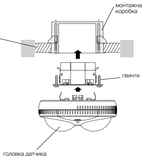
Схема установки / внутрішній монтаж
