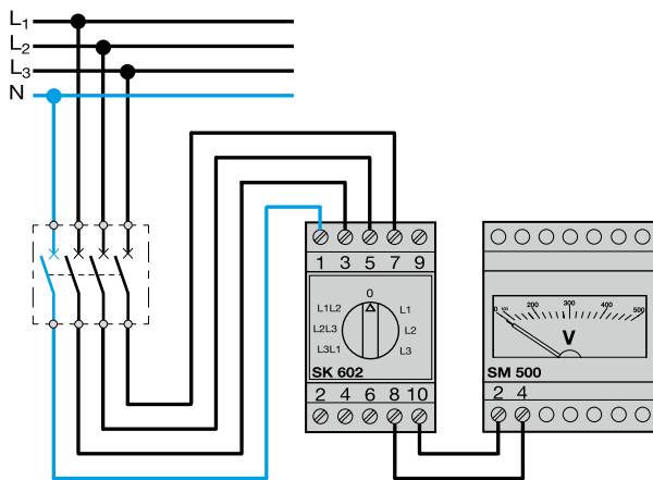
Електричне підключення вольметра з перемикачем SK602
