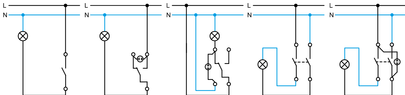
Вимикач однополюсний
