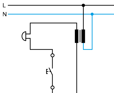
Управління квартирним дзвінком за допомогою кнопки серії 1/0 (Неонові лампочки не вставляються)
