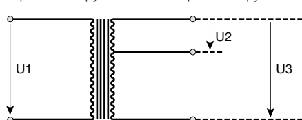
первинна напруга
