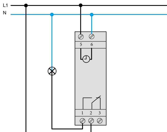
Схеми електричних з'єднань EG010, EG071
