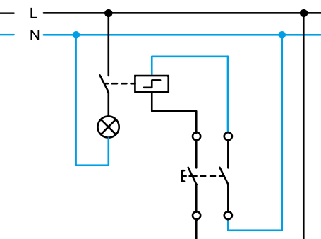
Включення освітлення за допомогою імпульсного реле, керованого двоклапотною кнопкою
