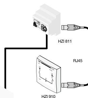
Підключення
