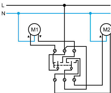
Управління жалюзі за допомогою поворотного перемикача (з фіксацією) з мех. блокуванням (схема при використанні клапового перемикача без фіксації аналогічна)
