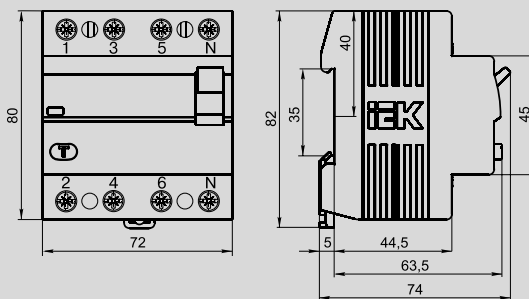
ВД1-63 4-полюсний
